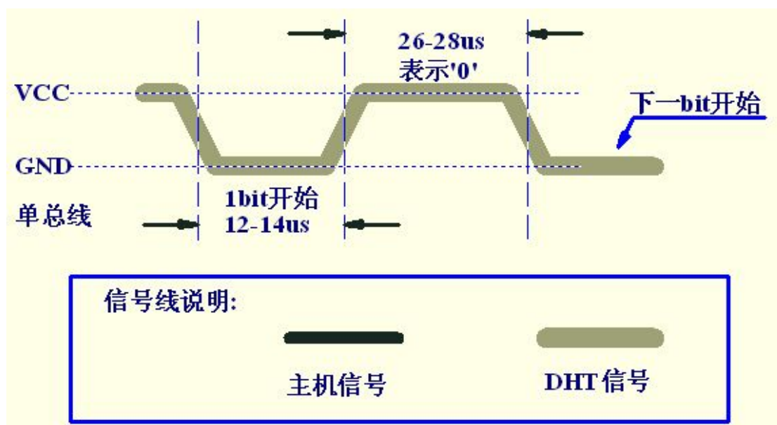
图7.3 信号‘0’时序图
