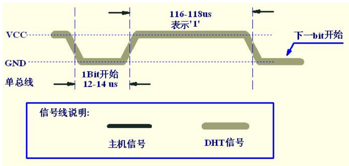
图7.4 信号‘1’时序图
