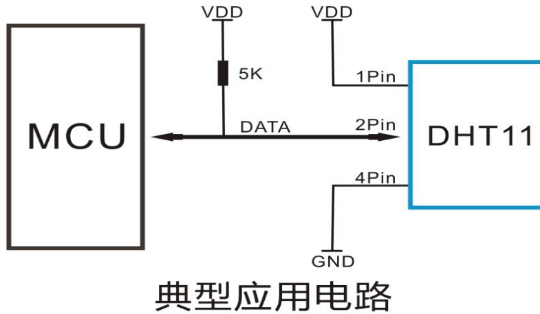
图5.0 典型电路连接
